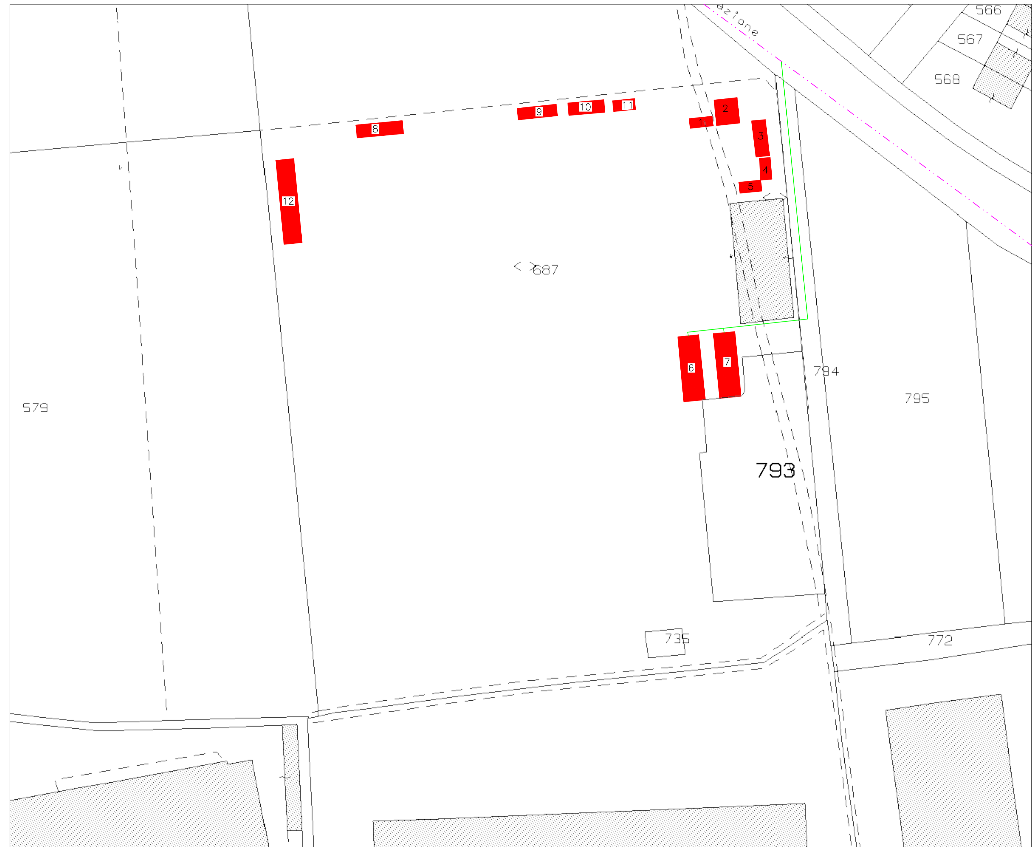
UBICAZIONE PREFABBRICATI E SCHEMA FOGNATURE
